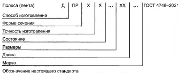
Рисунок 1 — Схема условного обозначения полос и лент
